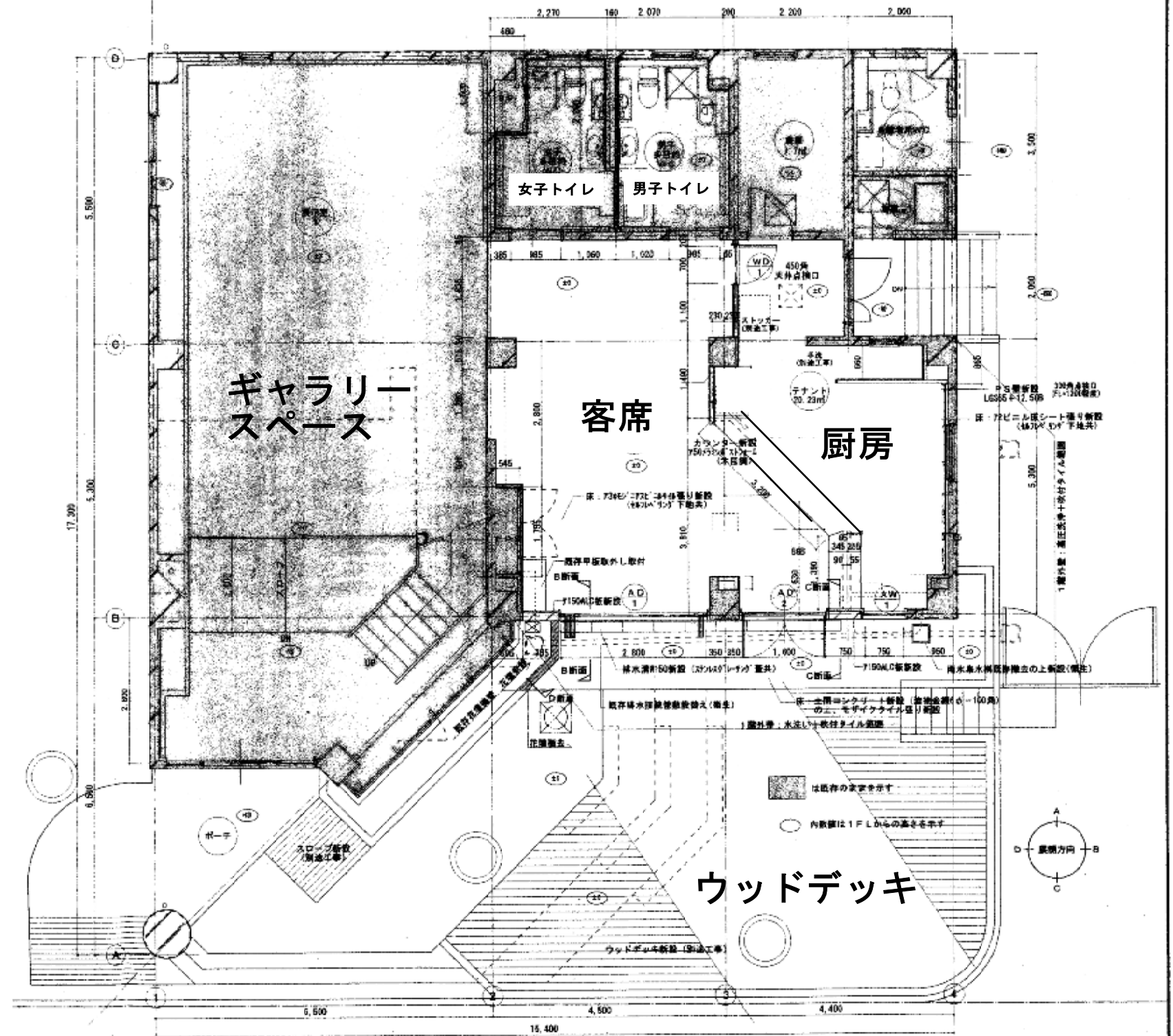
1階 改修後平面詳細図 縮尺1/50
